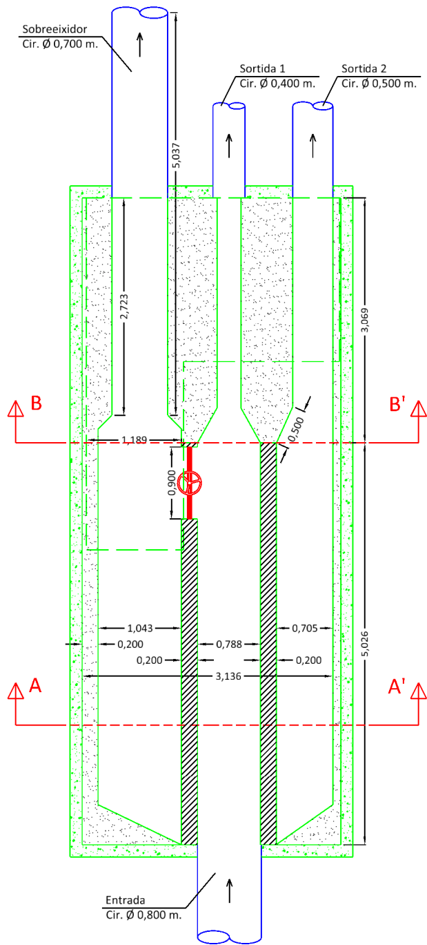
Planta Registre Sifó Goya
