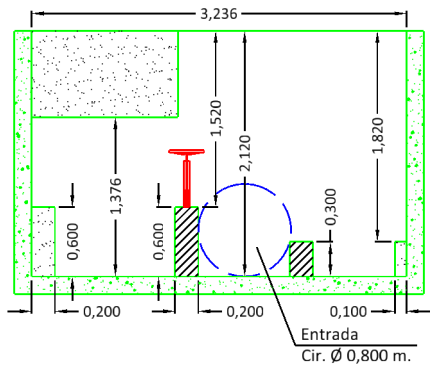
Perfil B-B' Registre Sifó Goya
