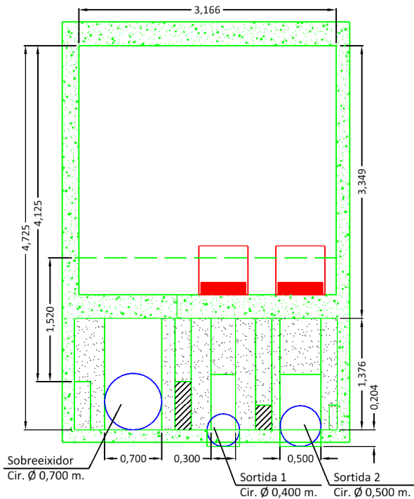
Perfil B-B' Registre Sifó Goya
