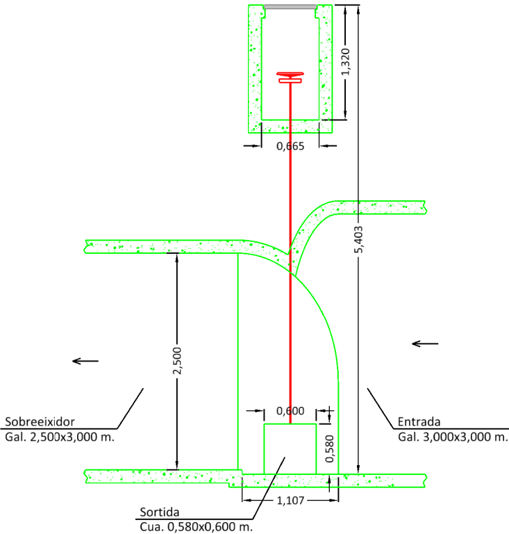
Perfil A-A' Sobreeixidor S10f
